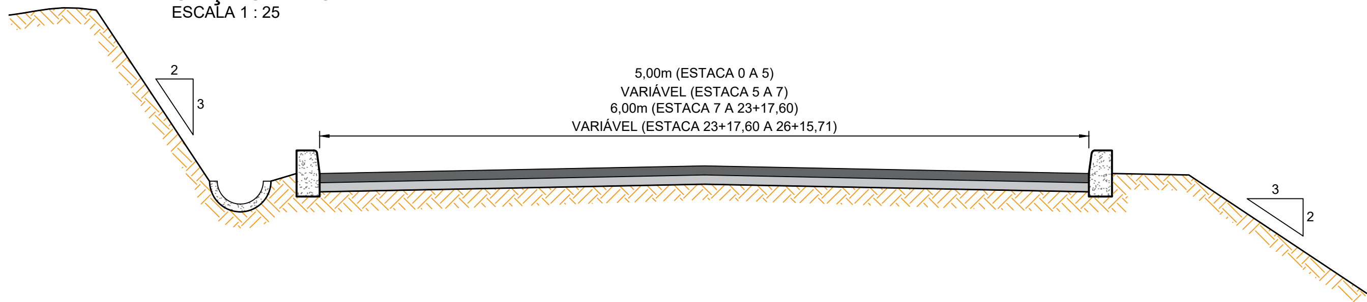
SEÇÃO TIPO ESCALA 1 : 25
